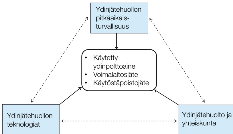
Kuva 2. KYT2018-tutkimusohjelman aihepiirit.
